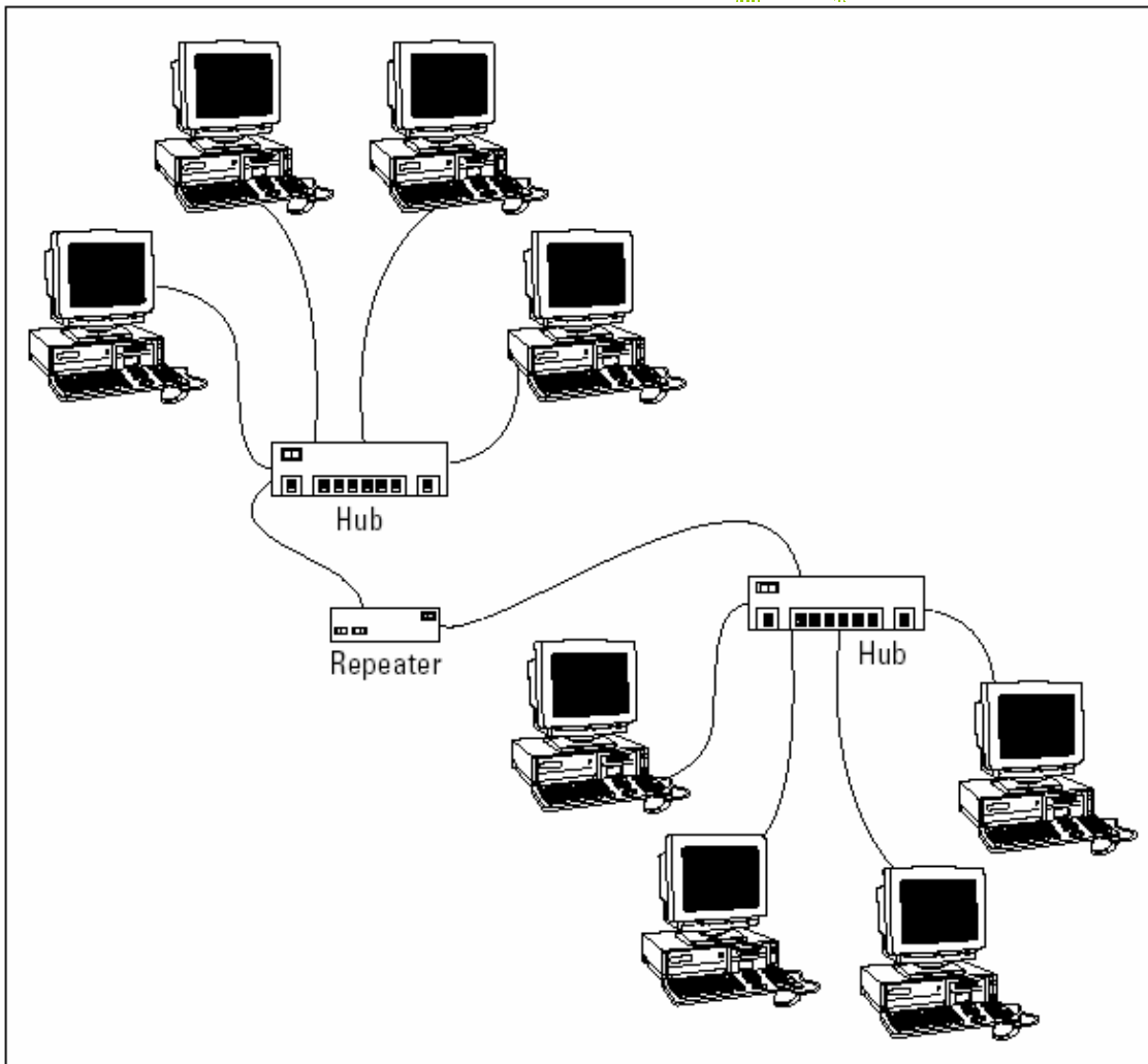
شکل ۳-۴ استفاده از تکرار کننده
